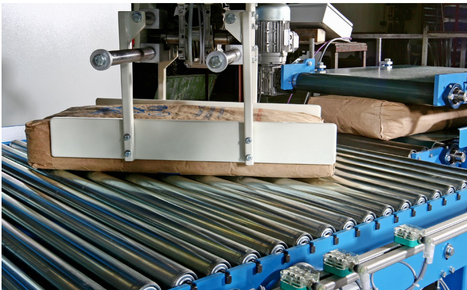
Greifer für Sackwaren mit vorgelagertem Pressband zur Egalisierung der Säcke
