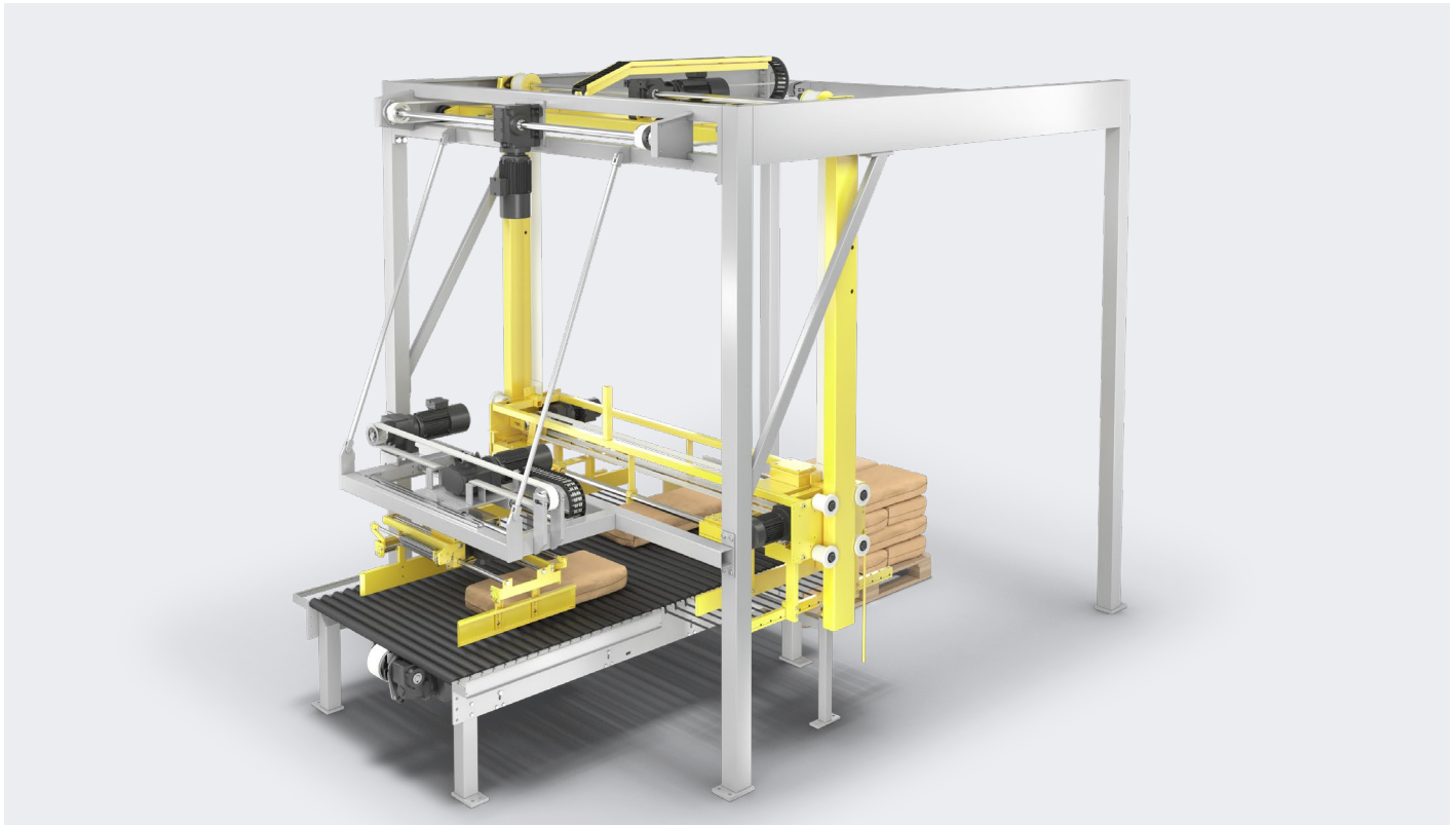
Palettierung von Sackwaren, der jeweils dritte Sack wird vor der Palettierung durch den Greifer passend gedreht
